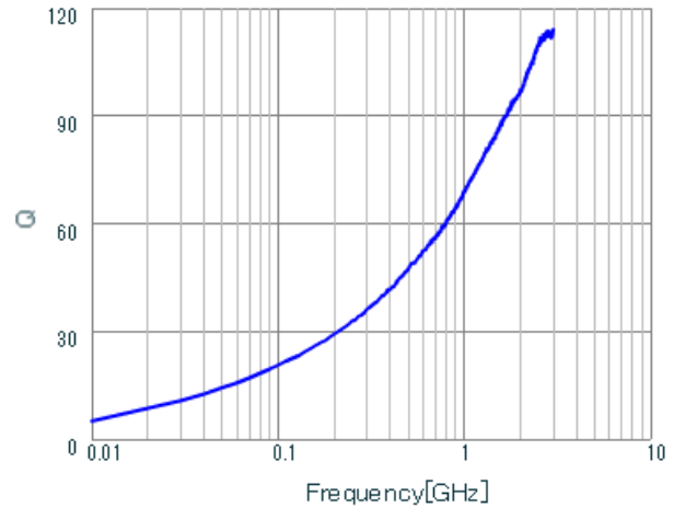
LQW18AN3N6D0Z Q.
