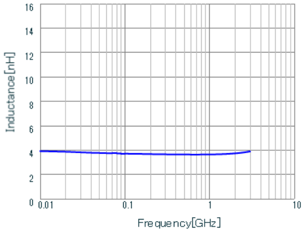
LQW18AN3N6D0Z L.
