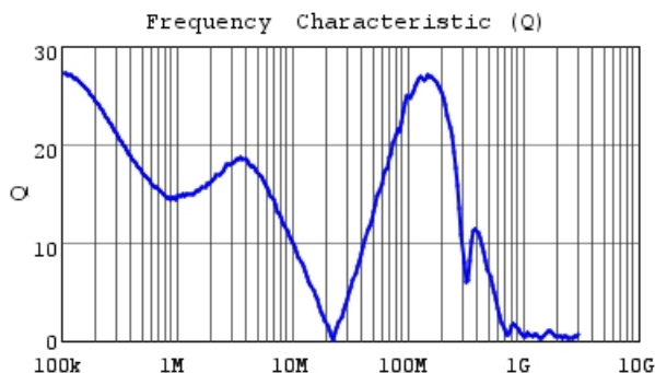
1253AY-220M Q
