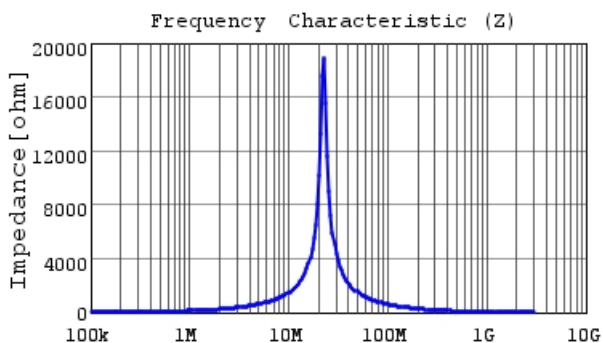
1253AY-220M |Z|
