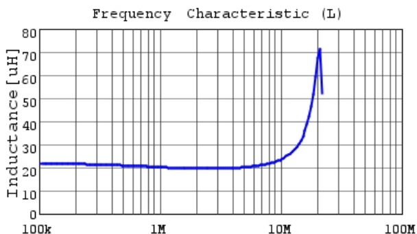
1253AY-220M L
