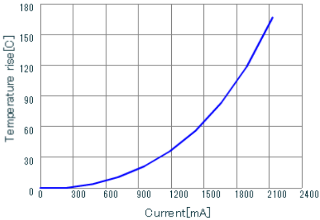
LQH3NPN100MGR DT_Current
