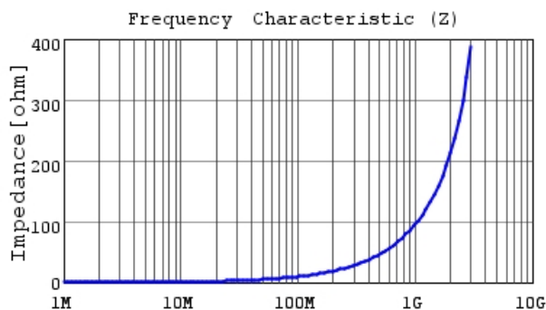
LQW15AN15NJ8Z |Z|
