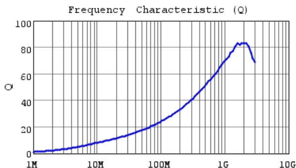
LQW15AN15NJ8Z Q
