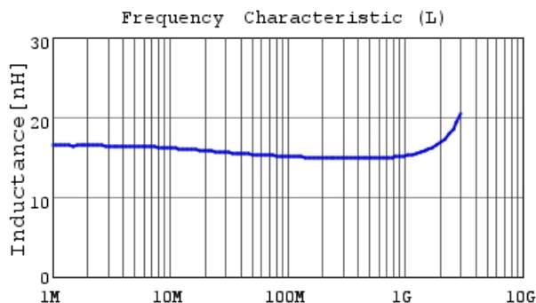
LQW15AN15NJ8Z L
