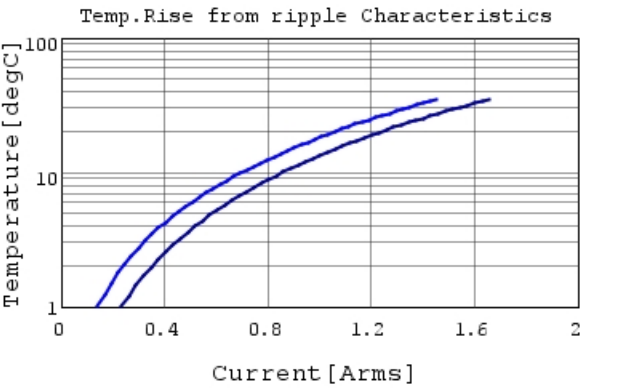
GRT033R61A224KE01 Temp.rise — 600kHz —
