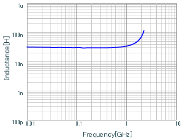
LQG15WH30NG02 L.
