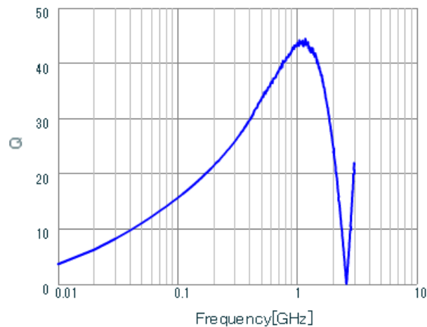
LQG15WH30NG02 Q.
