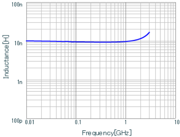
LQG15WZ9N5G02 L.
