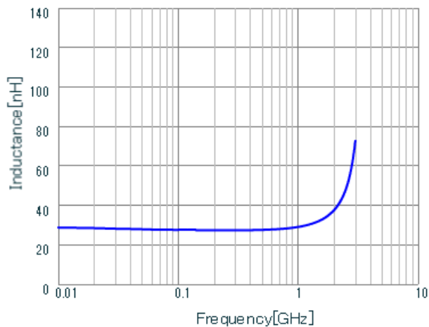
LQW18AN27NG0Z L.
