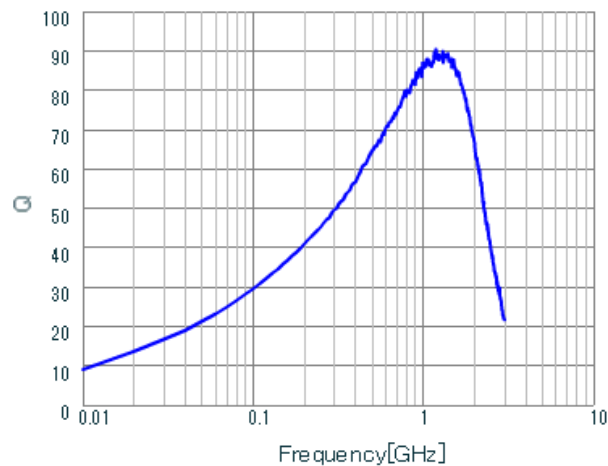
LQW18AN27NG0Z Q.
