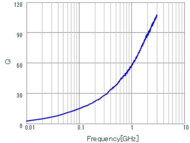
LQG15HN1N2S02 Q.
