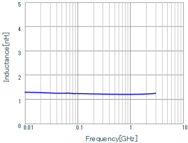
LQG15HN1N2S02 L.
