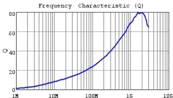
LQW15AN18NJ80 Q
