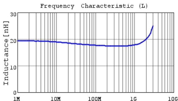
LQW15AN18NJ80 L
