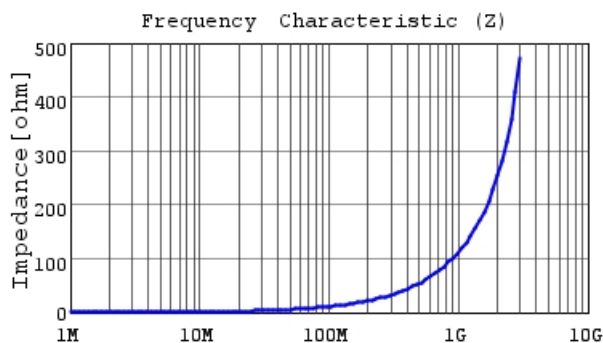
LQW15AN18NJ80 |Z|
