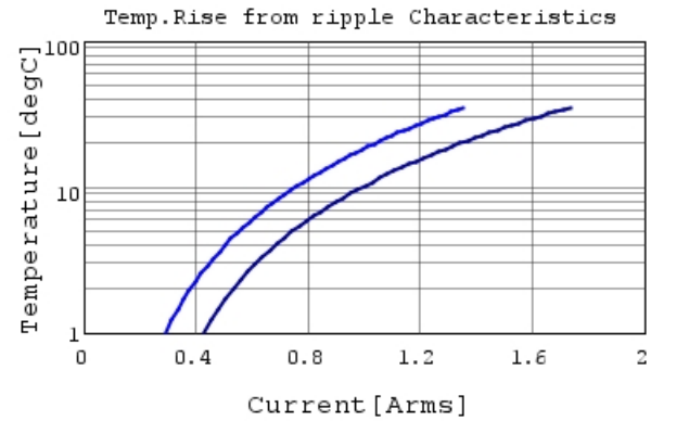
GRM155C80G224KE01 Temp.rise — 500kHz —
