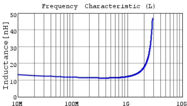
LQG15HH12NJ02 L
