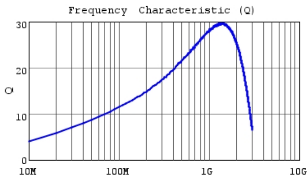
LQG15HH12NJ02 Q
