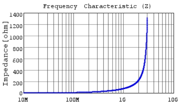
LQG15HH12NJ02 |Z|
