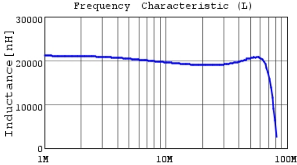
LQW32FT220M0H L
