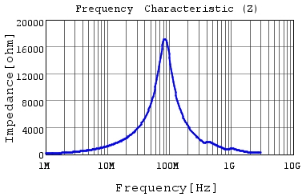
LQW32FT220M0H |Z|
