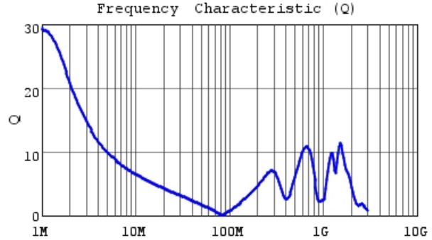
LQW32FT220M0H Q
