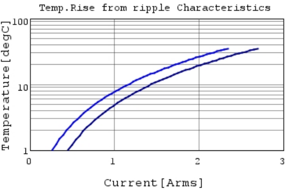
GRT033R60J105ME13 Temp.rise 500kHz
