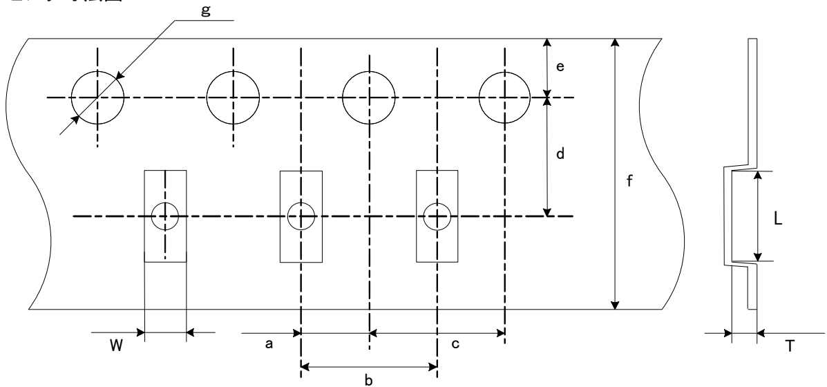
テーピング寸法図
