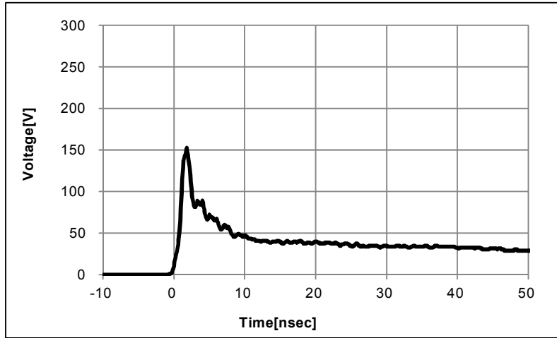
ESD 波形 (IEC61000-4-2:8kV 接触条件)
