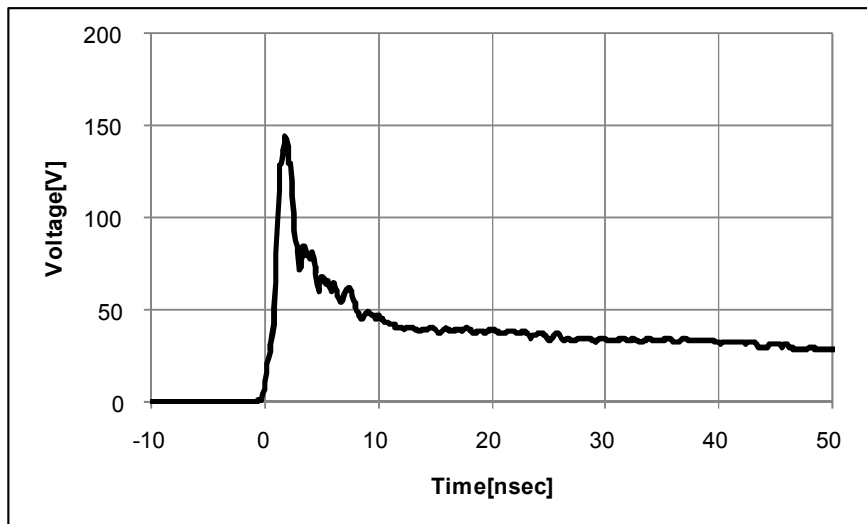
ESD 波形 (IEC61000-4-2:8kV 接触条件)
