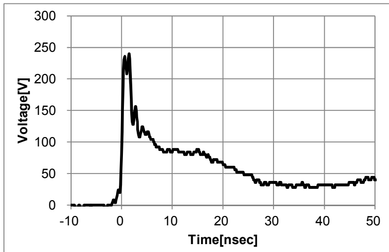
ESD 波形 (IEC61000-4-2:8kV 接触条件)
