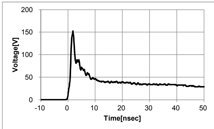
ESD 波形 (IEC61000-4-2:8kV 接触条件)
