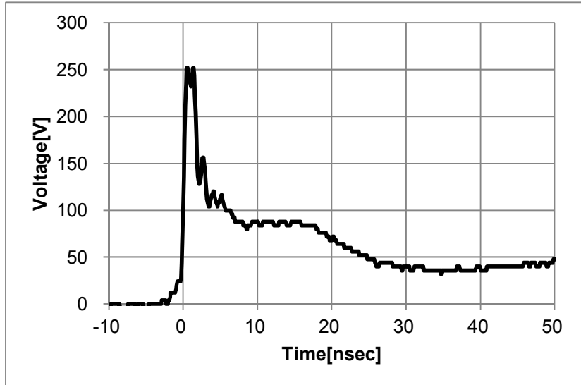
ESD 波形 (IEC61000-4-2:8kV 接触条件)
