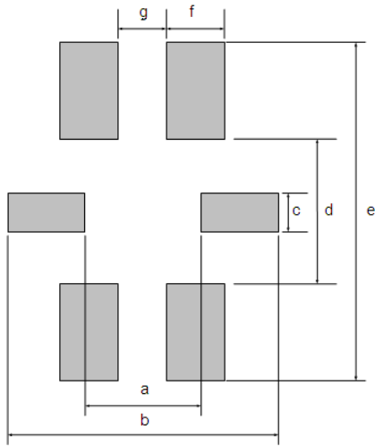
付図.1 推奨ランドパターン LXES11D series
