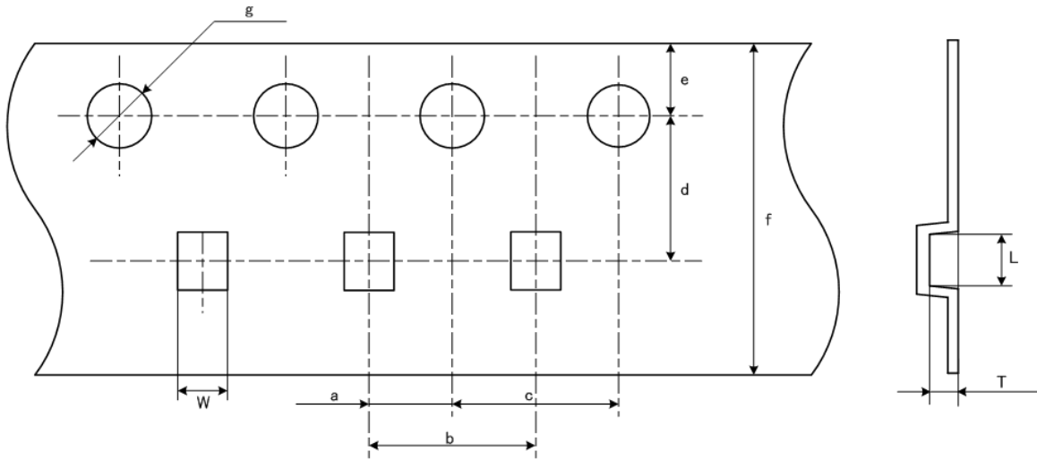
テーピング寸法図
