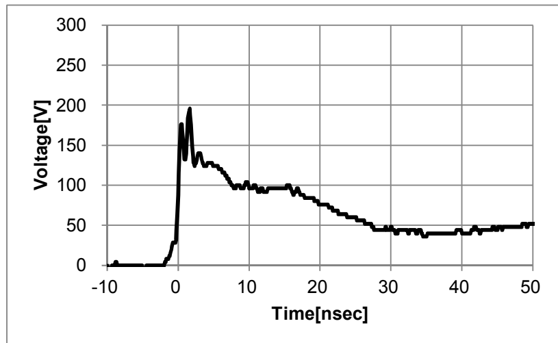
ESD 波形 (IEC61000-4-2:8kV 接触条件)
