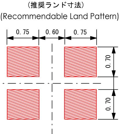
第1図 外形寸法図 Figure 1. Dimensions
