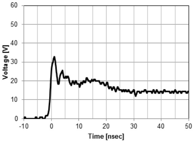
ESD 波形(IEC61000-4-2:8kV 接触条件)
