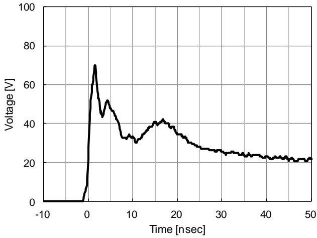
ESD 波形(IEC61000-4-2:8kV 接触条件)
