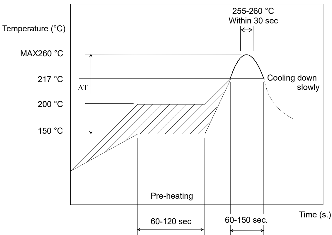
リフローはんだ付け条件
