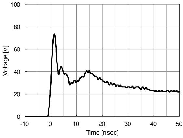
ESD 波形(IEC61000-4-2:8kV 接触条件)
